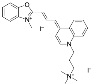
Struktur von YO-TAP-3
