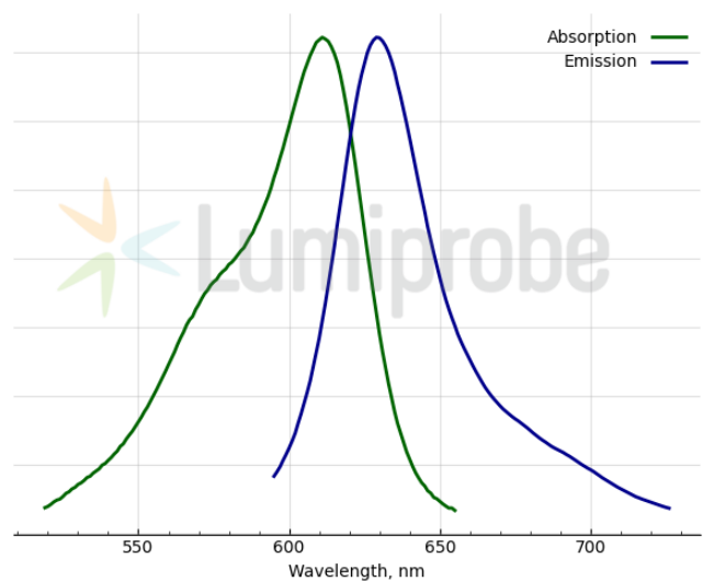
Absorptions- und Emissionsspektren von YO-TAP-3 (DNA-Farbstoff-Komplex)
