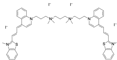
Struktur von TODi-3
