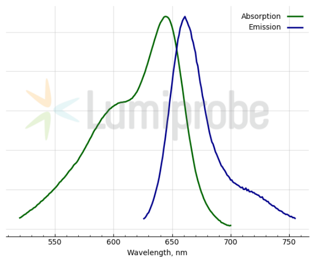
Absorptions- und Emissionsspektren von TODi-3 (DNA-Farbstoff-Komplex)
