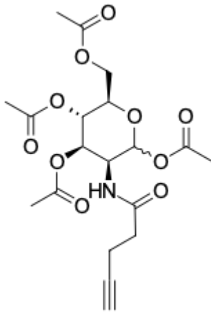
Struktur von Ac4ManNAI (N-(4-pentynoyl)-mannosamin-tetraacyliert)
