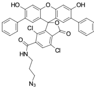
Struktur von SIMA-Azid, 6-Isomer
