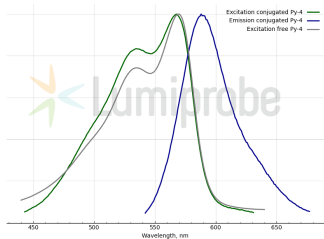
Anregungs- und Emissionsspektren von Pyrylium-4 (Py-4)
