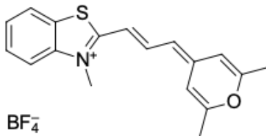
Struktur von Pyrylium-4 (Py-4)
