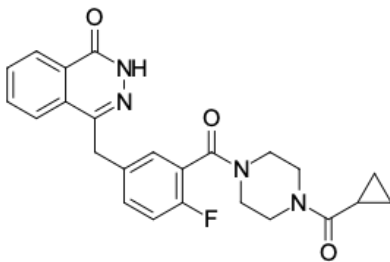
Struktur von Olaparib
