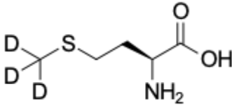
Struktur von L-Methionin (S-Methyl-d3)
