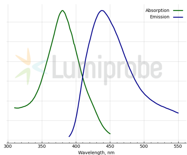
Absorptions- und Emissionsspektren von Hoechst 34580 (DNA-Farbstoff-Komplex)
