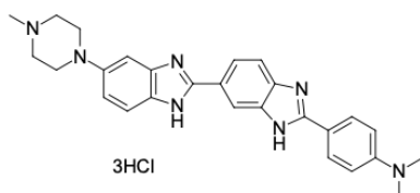
Struktur von Hoechst 34580
