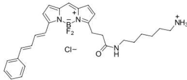
Struktur von BDP-581/591-amin
