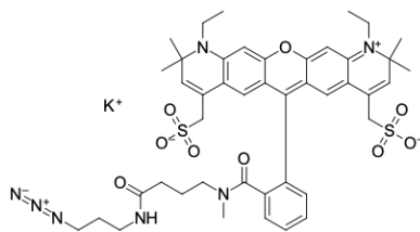
Struktur von ATT 594 Azid
