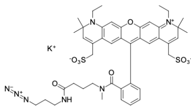
Struktur von ATT 594 Azid
