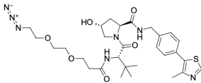
Struktur von (S,R,S)-AHPC-PEG2-C2-Azid
